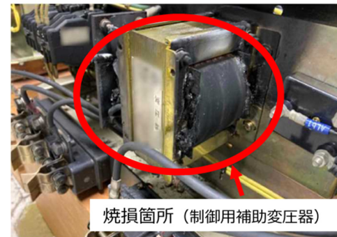
柏崎刈羽発電所の電源設備の 発煙発火は、公設消防が非火災 と判定(2025 年4月1日発生)
