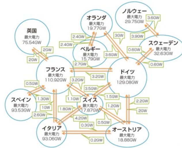
欧州は強固な送電系統で国家間の連系 出典:IEA Electricity Information 2010
